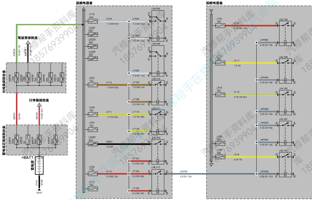
电源分布(1)
