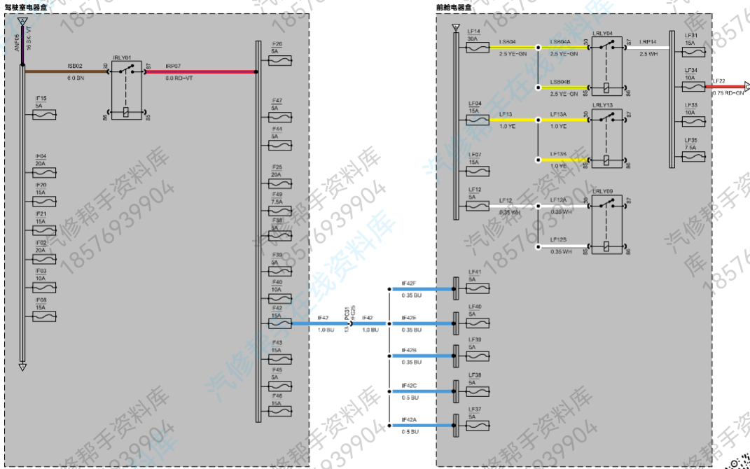
电源分布(2)
